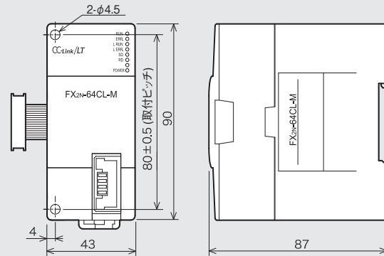
FX2N-64CL-M
