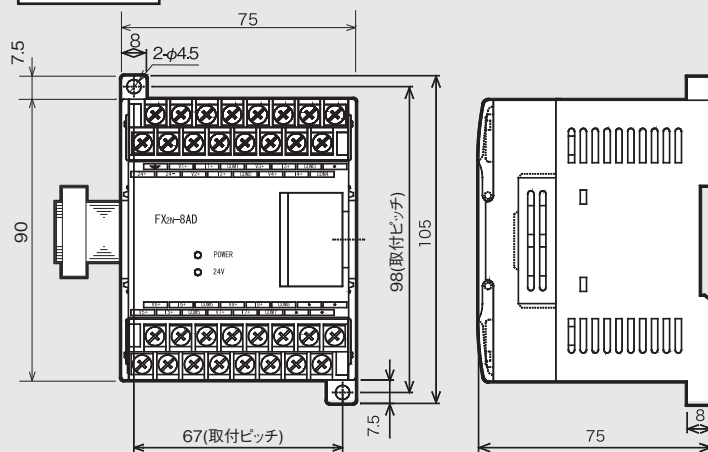
FX2N-8AD
