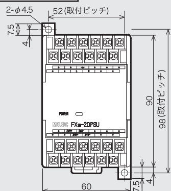
FX2N-20PSU 質量: 0.3kg
