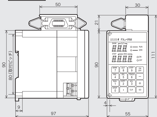
FX2N-1RM 質量: 0.5kg
