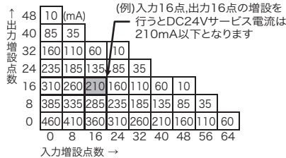
FX2N-48E(AC電源・DC入力タイプ)
