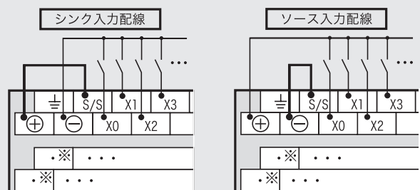
[DC電源タイプの入力配線図]
