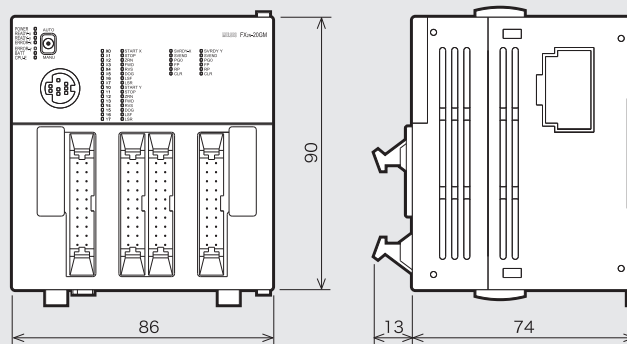
FX2N-20GM 質量: 0.4kg
