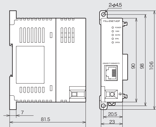
FX3U-ENET-ADP 質量: 0.1kg
