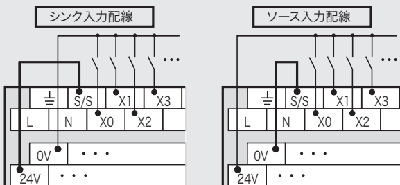
[AC電源タイプの入力配線図]
