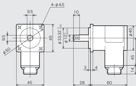
F2-720RSV 質量: 0.4kg
