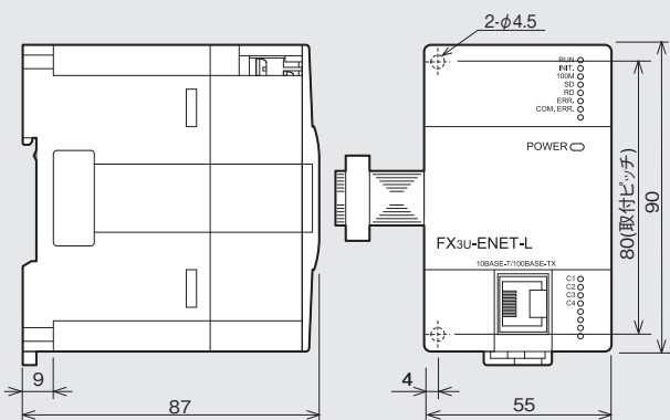
FX3U-ENET-L
