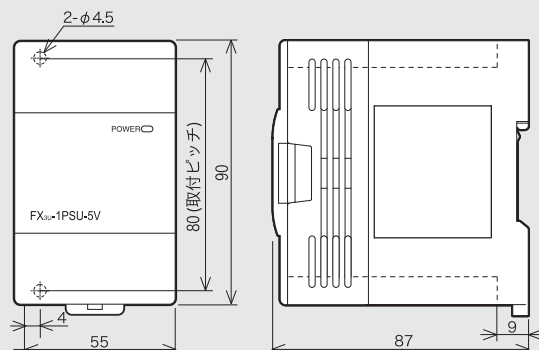
FX3U-1PSU-5V 質量: 0.3kg 外装色 マンセル 0.08GY/7.64/0.81 単位 mm
