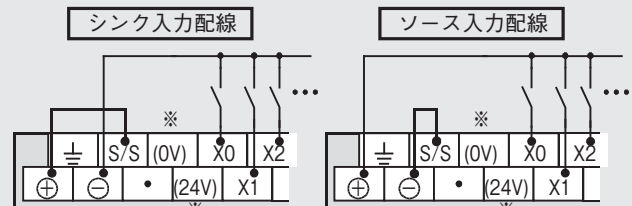
[DC電源タイプの入力配線図]
