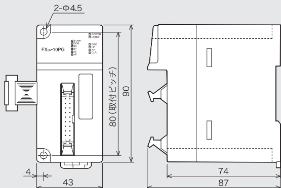
FX2N-10PG 質量: 0.2kg
