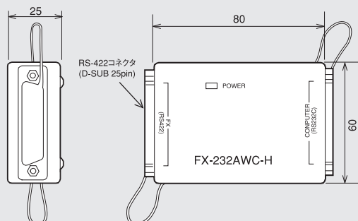
FX-232AWC-H 質量: 0.1kg
