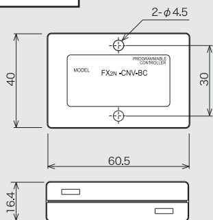
FX2N-CNV-BC 質量: 0.04kg
