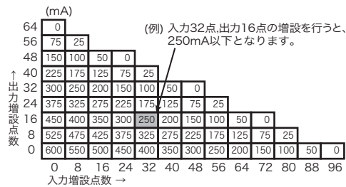
FX3U-48~128M
