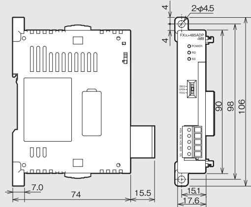
FX3U-485ADP(-MB) 質量: 0.08kg
