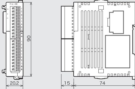
FX2NC-4AD
