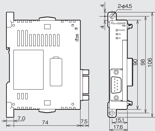
FX3U-232ADP(-MB) 質量: 0.08kg
