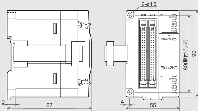
FX3U-2HC
