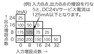
FX2N-48E
