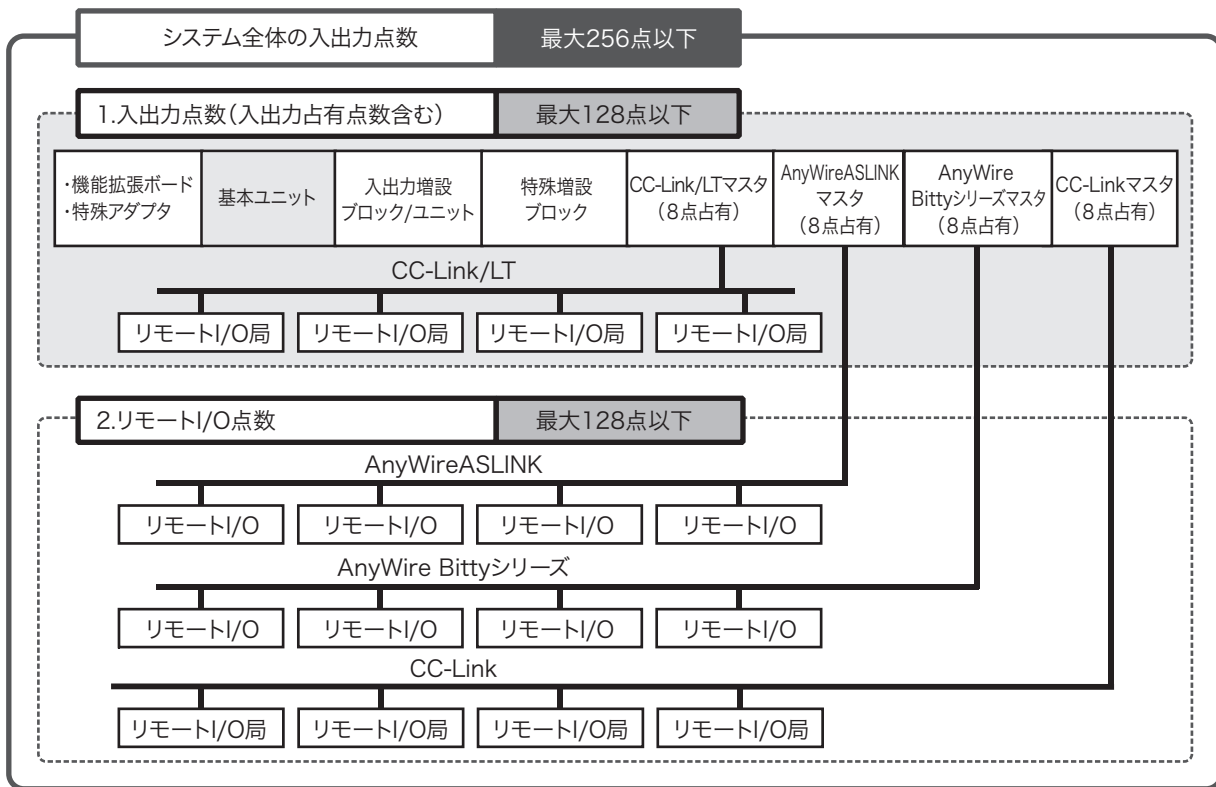
[ネットワーク マスタ接続時の概念図]
