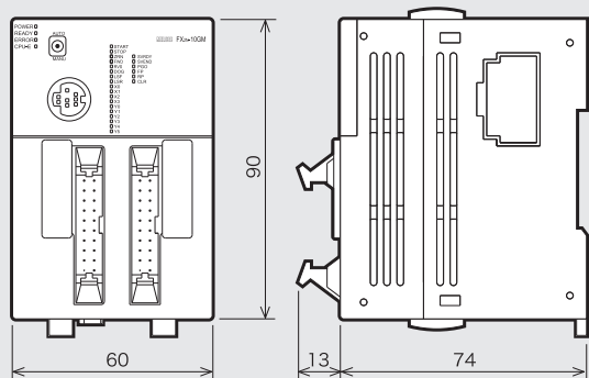
FX2N-10GM 質量: 0.3kg
