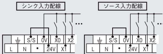
[AC電源タイプの入力配線図]
