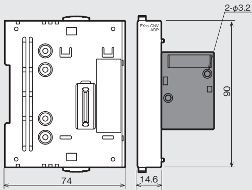
FX3s-CNV-ADP 質量: 0.1kg
