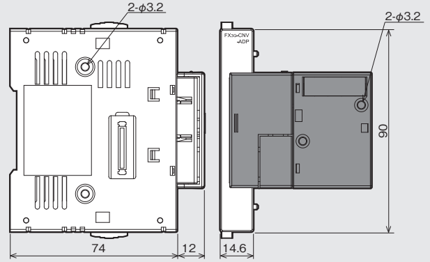
FX3G-CNV-ADP 質量: 0.1kg
