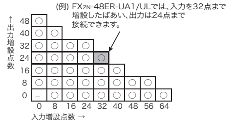
FX2N-48ER-UA1/UL(AC電源・AC入力タイプ)
